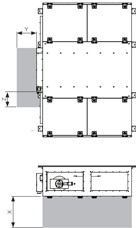
Abb. 10-6 Mindestabstand für Wartungsarbeiten
