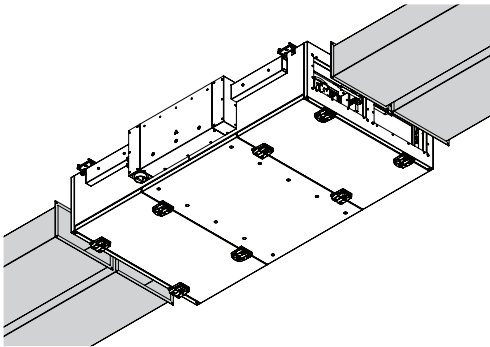
Abb. 10-7 Anschluss Luftkanal
