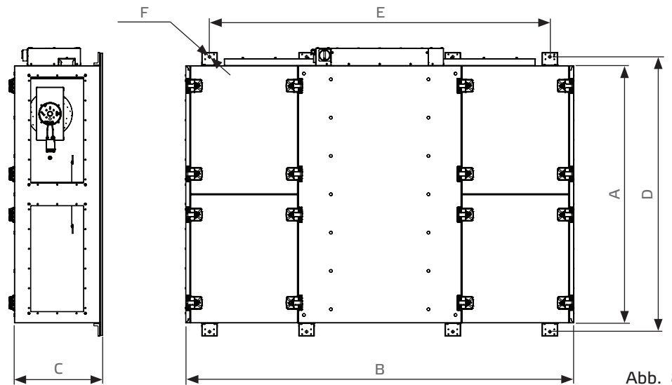
Abb. 8-1 Abmessungen des Gerätes
