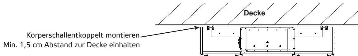
Abb. 10-2 Deckenmontage
