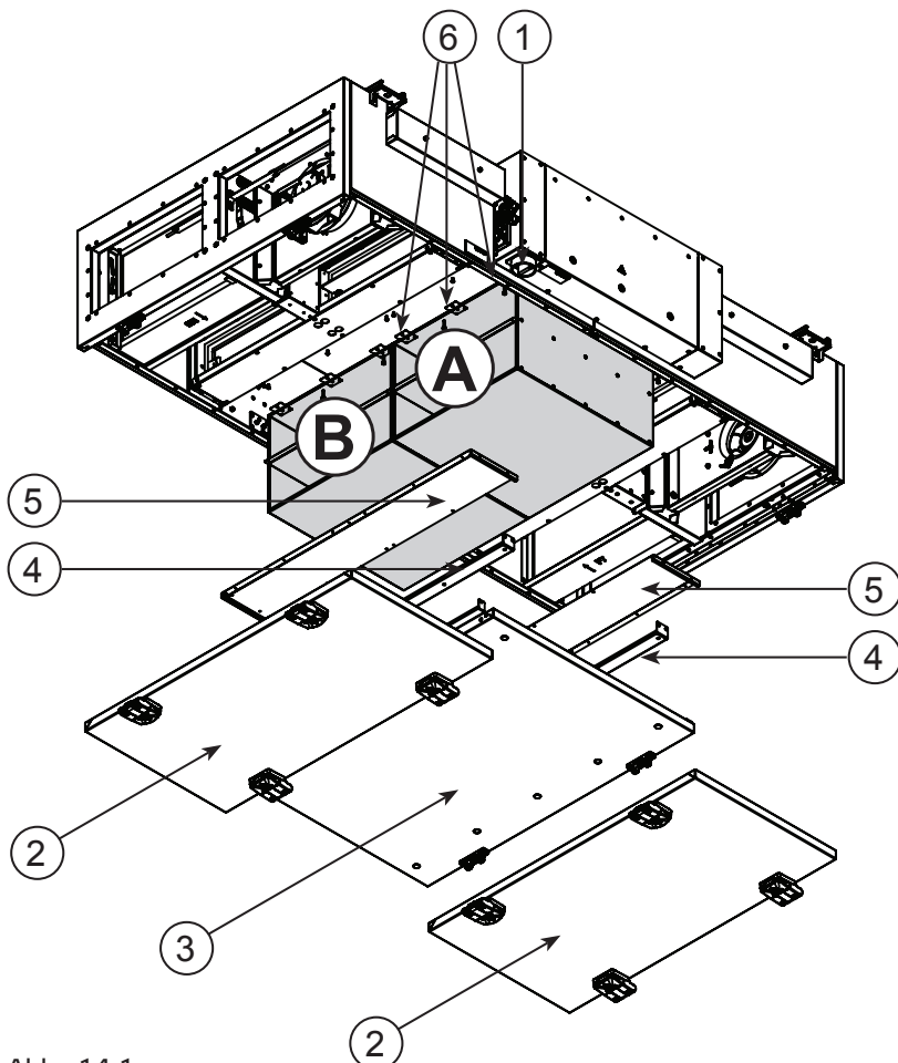
Abb. 14-1 Ausbau Speichermassenwärmetauscher
