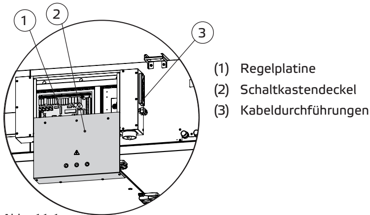
Abb. 11-1 Anschlussraum
