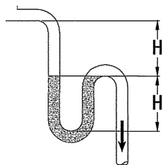
Abb. 10-7 Sperrwasserhöhe H
