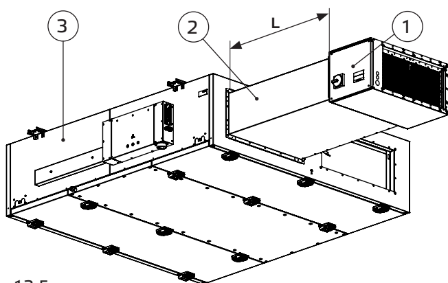
Abb. 13-5 Anschluss EHM an Gerät
