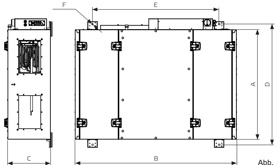
Abb. 8-1 Abmessungen des Gerätes
