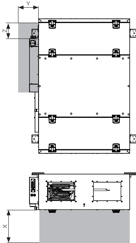
Abb. 10-2 Mindestabstand für Wartungsarbeiten
