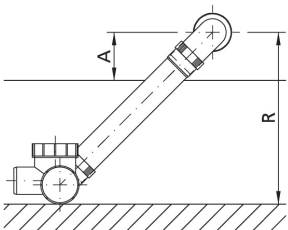
Abb. 10-10 Ermittlung Grundrahmenhöhe GR
