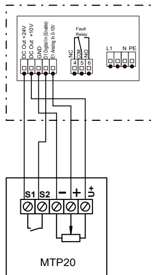
Anschluss Potentiometer MTP20
