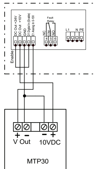
Anschluss Potentiometer MTP30
