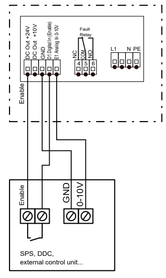
Anschluss 0-10V Signal
