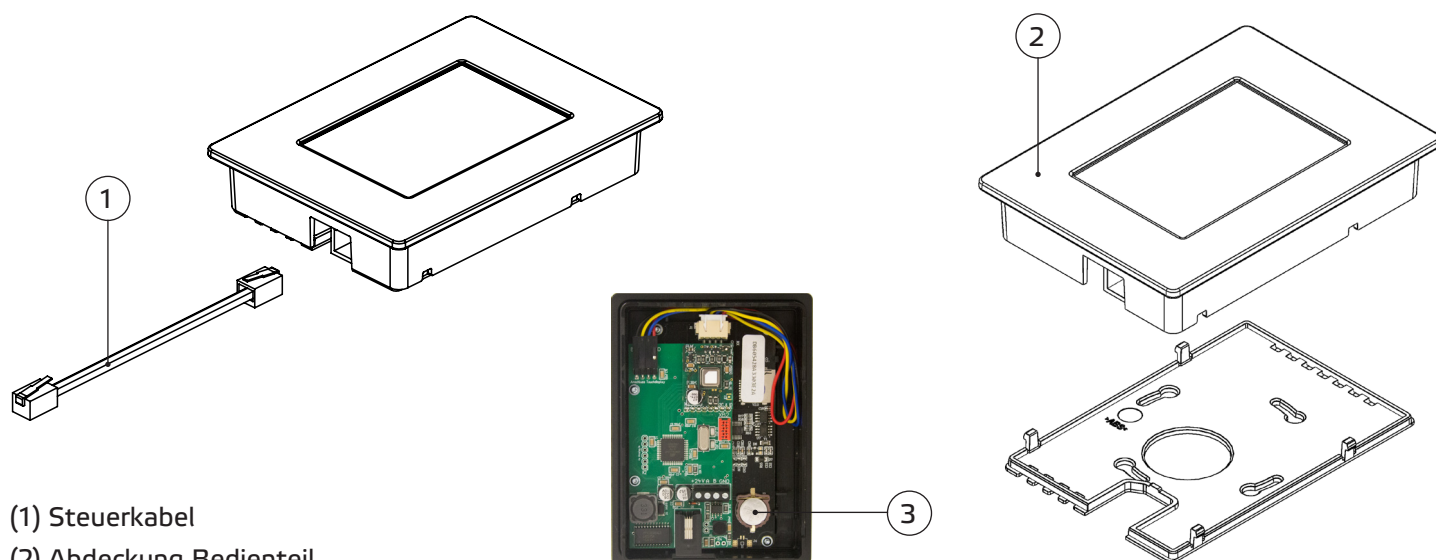
Abb. 14-8 Batteriewechsel Bedienteil
