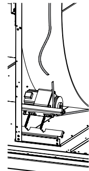
Abb. 14-2 Entfernen des defekten Antriebsriemens.
