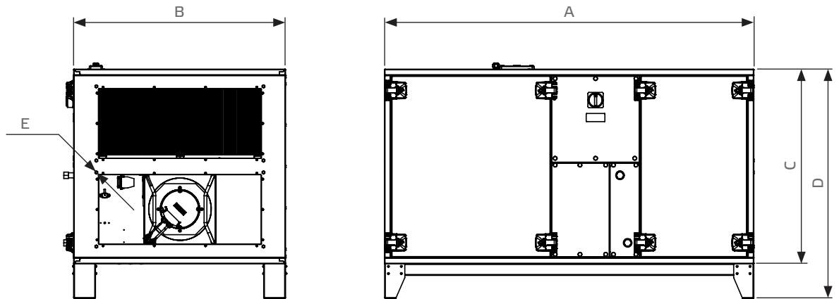
Abb. 8-1 Abmessungen des Gerätes
