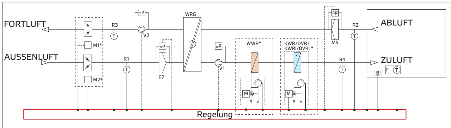
Abb. 13-2 Anschlussschema
