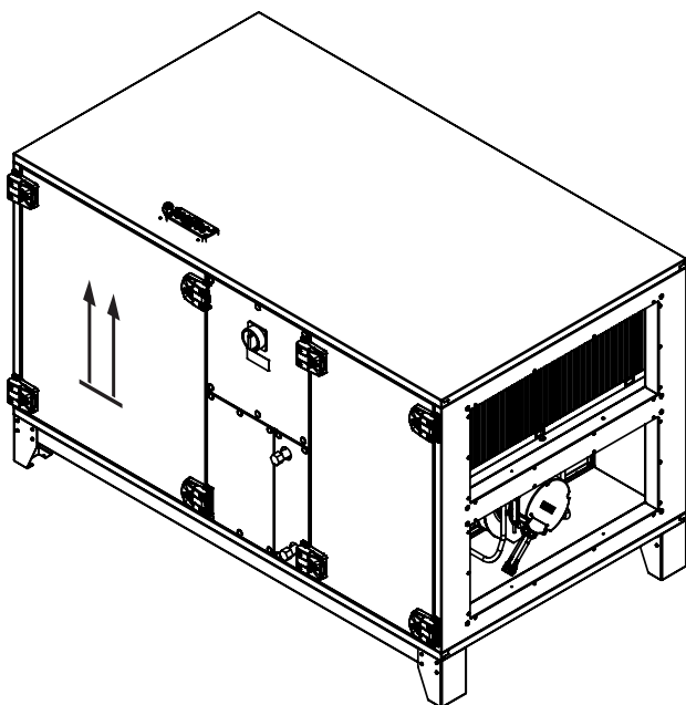
Abb. 10-1 Erlaubte Einbaulage
