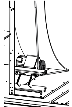
Abb. 14-5 Auf einwandfreien Lauf des Riemens auf der Riemenscheibe ist zu achten.
