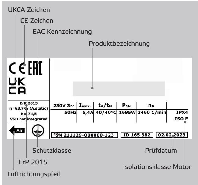
Abb. 5-6 Typenschild
