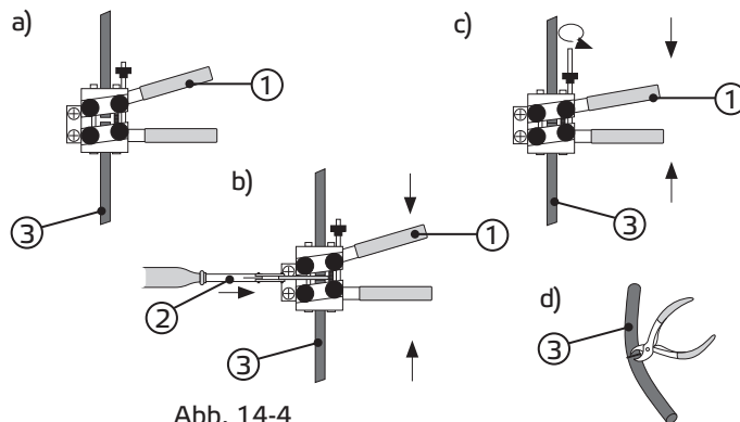
Abb. 14-4 Verschweißen des Antriebsriemens (3) mit Klemme (1) und Schweiß-Spiegel (2).
