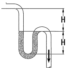
Abb. 10-13 Sperrwasserhöhe H
