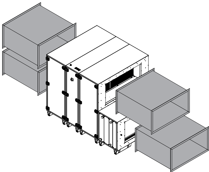
Abb. 10-9 Anschluss Luftkanal
