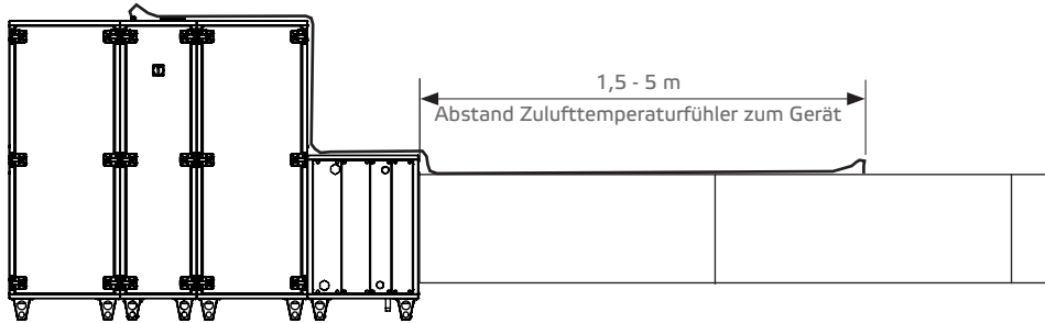
Abb. 10-7 Mindestabstand Zulufttemperaturfühler
