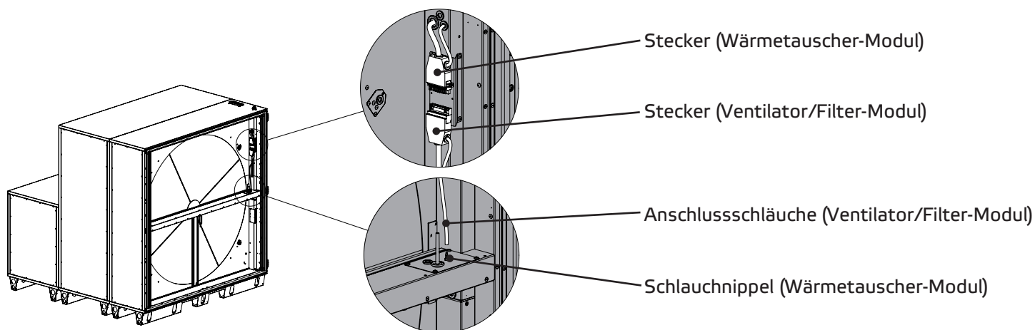
Abb. 10-6 Beschreibung Modulverbindungen 4
