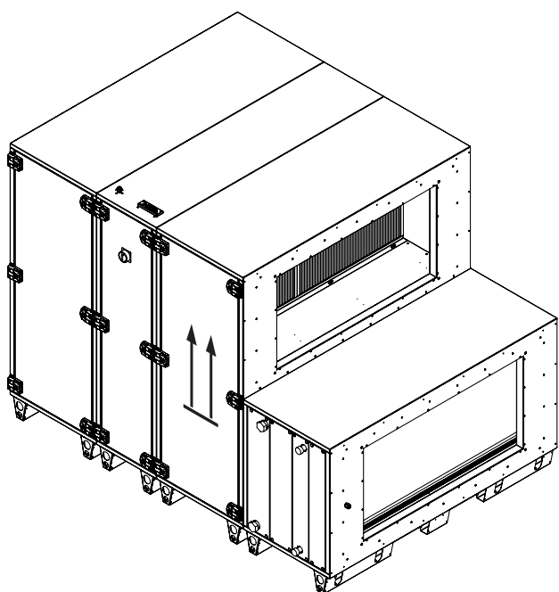
Abb. 10-1 Erlaubte Einbaulage
