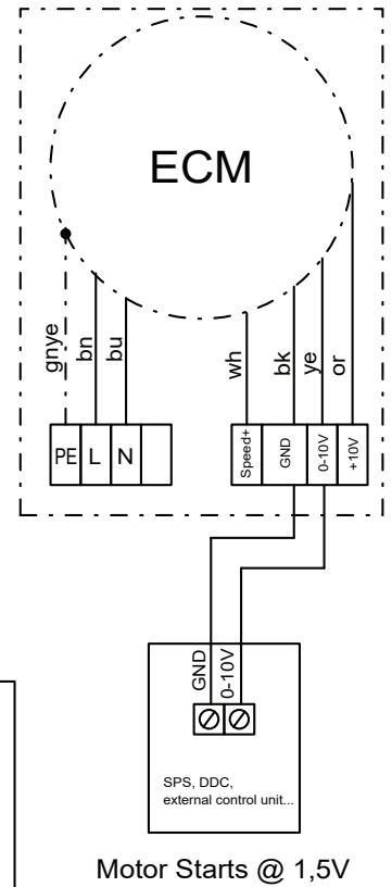
Anschluss 0-10V Signal
