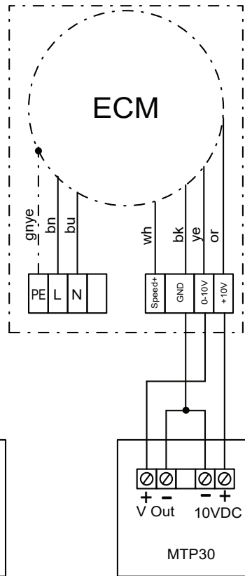
Anschluss Potentiometer MTP30
