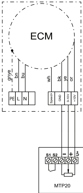
Anschluss Potentiometer MTP20
