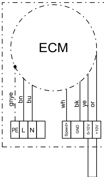
Keine Drehzahlregelung 100% Leistung
