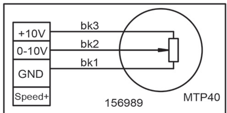
Anschluss mit beiliegendem Potentiometer
