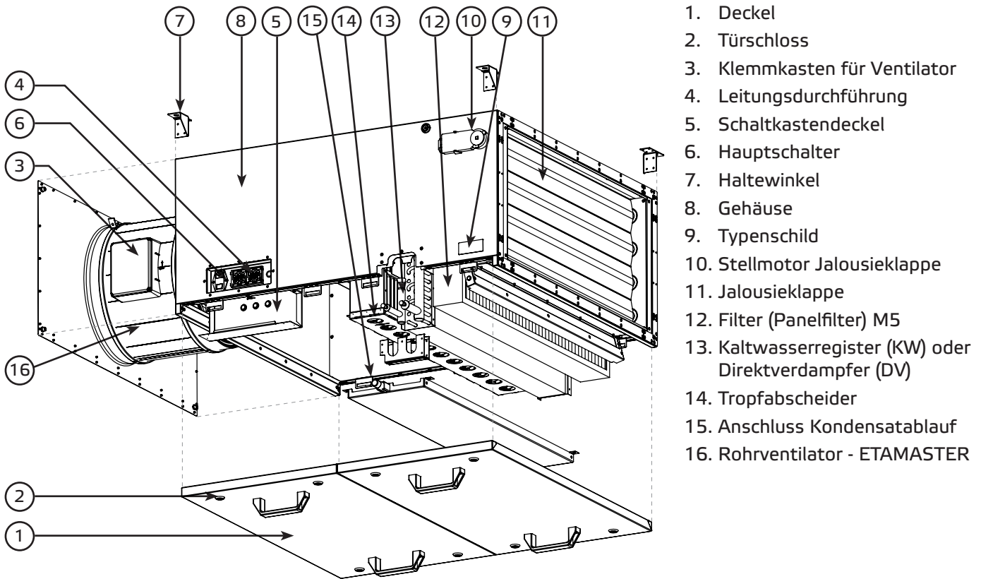
Abb. 5-3 SL...F OD
