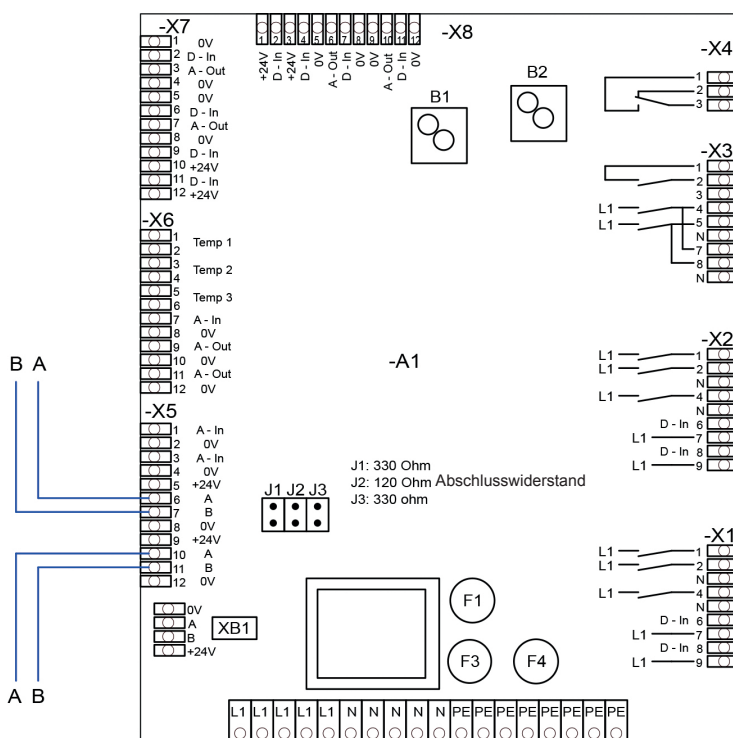
Abb. 15-1 Anschlussplan ModBus
