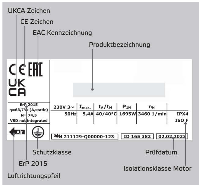
Abb. 5-3 Typenschild
