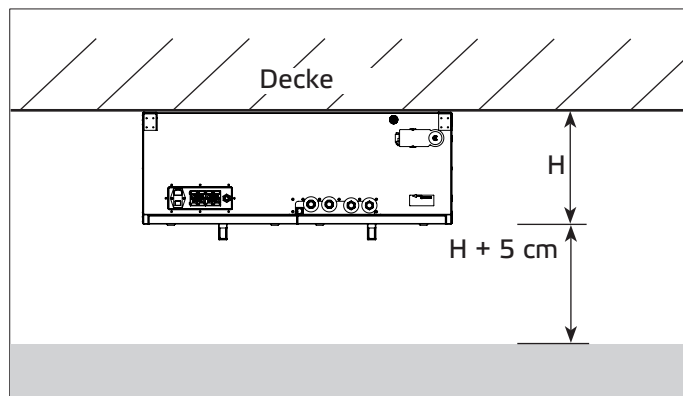
Abb. 10-3 Mindestabstand für Wartungsarbeiten
