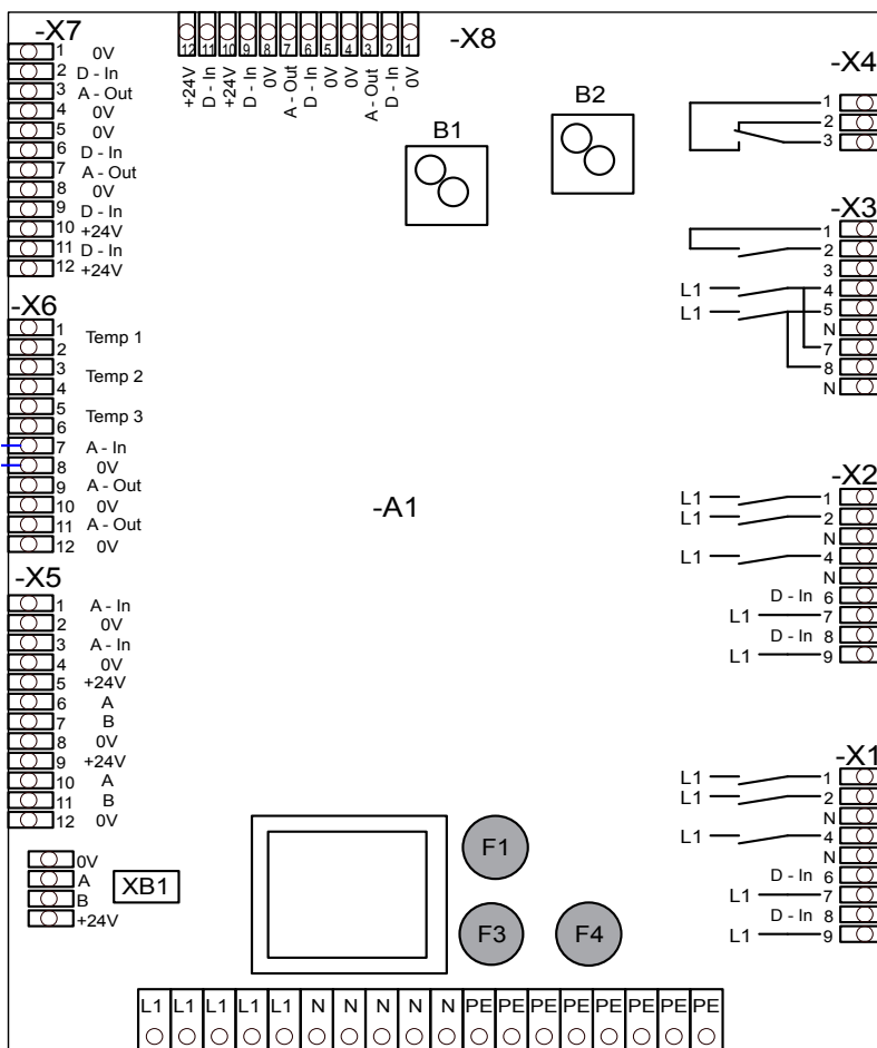
Abb. 18-1 Platine mit Feinsicherungen F1.
