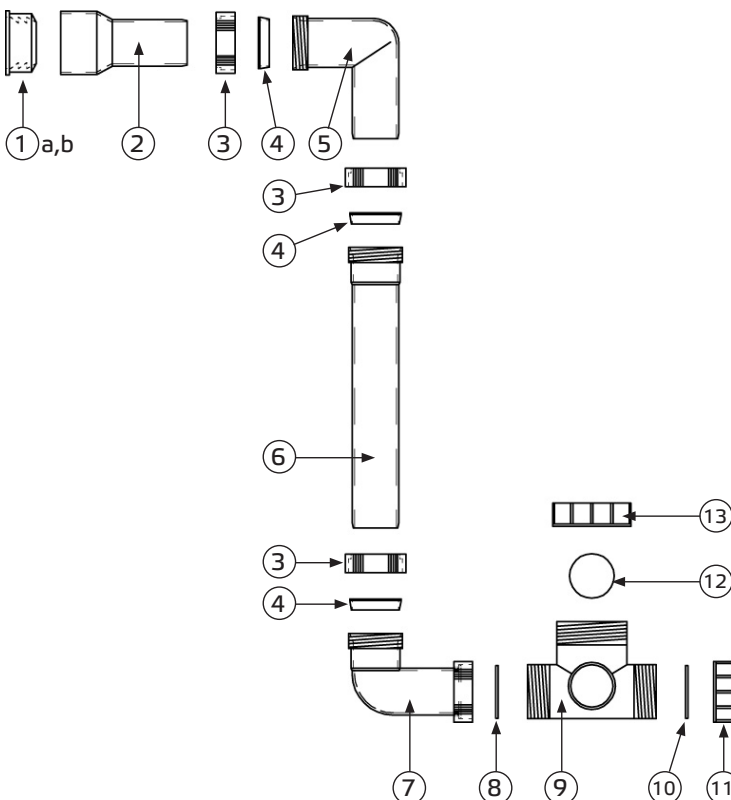
Abb. 10-8 Systemskizze Kugelsiphon SYS 02
