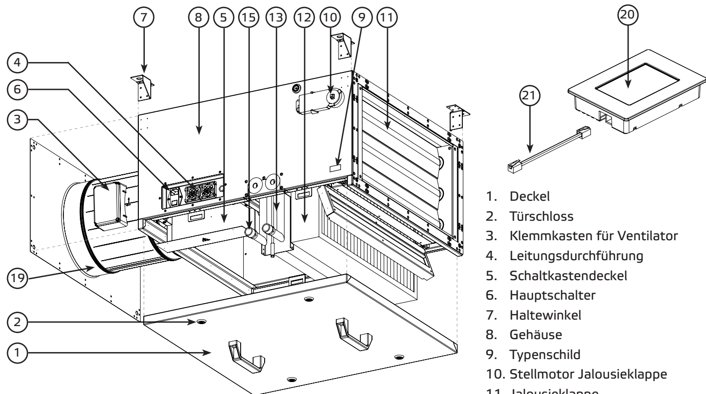
Abb. 5-1 SL...F WO
