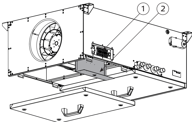
Abb. 11-1 (1) Kabledurchführungen
