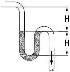
Abb. 10-7 Sperrwasserhöhe H
