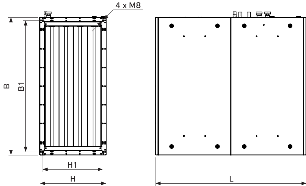
Abb. 8-1 Abmessungen des Gerätes
