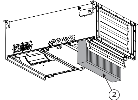
Abb. 14-2 Luftfilter herausnehmen und austauschen! (2) = Panelfilter M5
