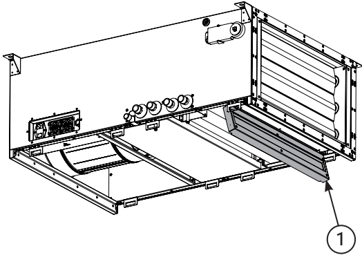
Abb. 14-1 (1) Luftfilterklappe lösen.
