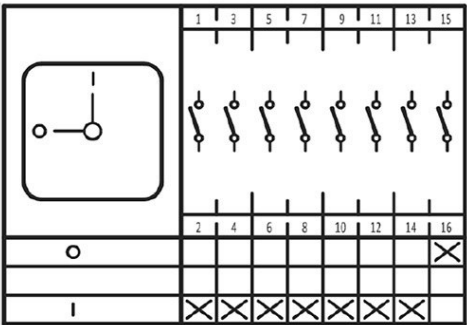
Schaltplan:
