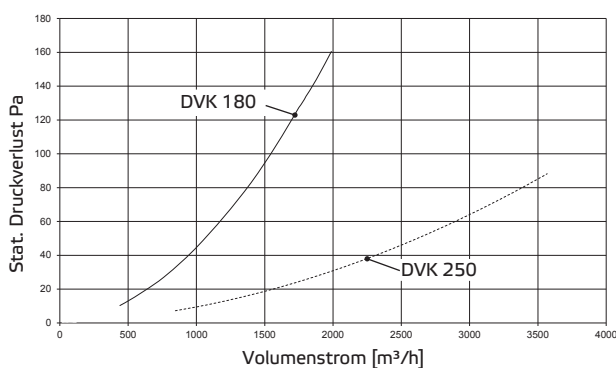
Druckverlustkennlinie (Dichte 1,2 kg/m³)
